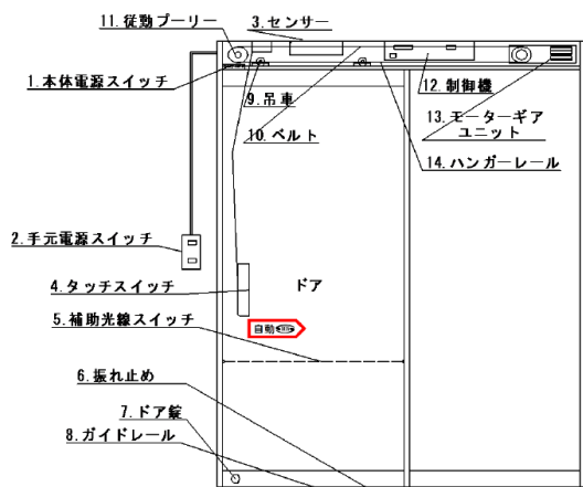
自動ドアエンジン装置の各部名称
